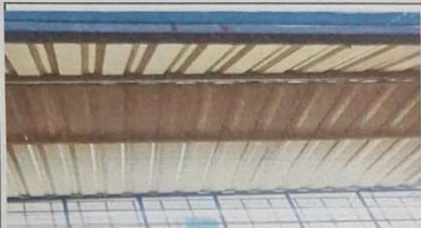
Foto1: Sustitución de lámina por lámina troquelada Aluzinc calibre 26 aula ubicada en el módulo 2 del establecimiento.
